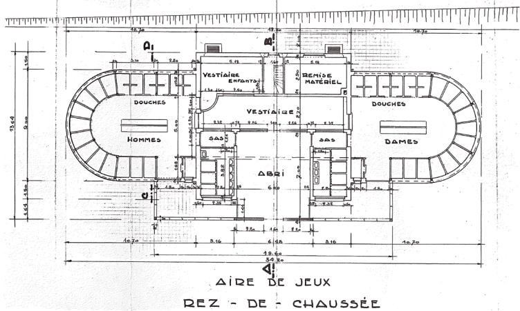
Plan. Projet 1950.
